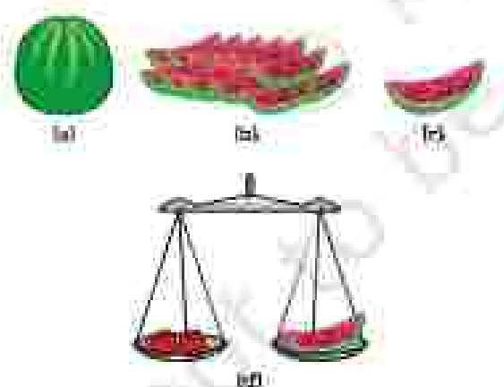
Fig. 3.4 : (a) Watermelon, (b) 12 pieces, (c) 1/12 of watermelon, (d) how the fruit seller can weigh the fruits using pieces of watermelon.
